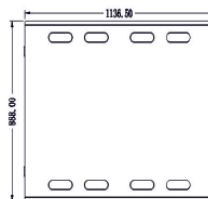
Вид сверху
